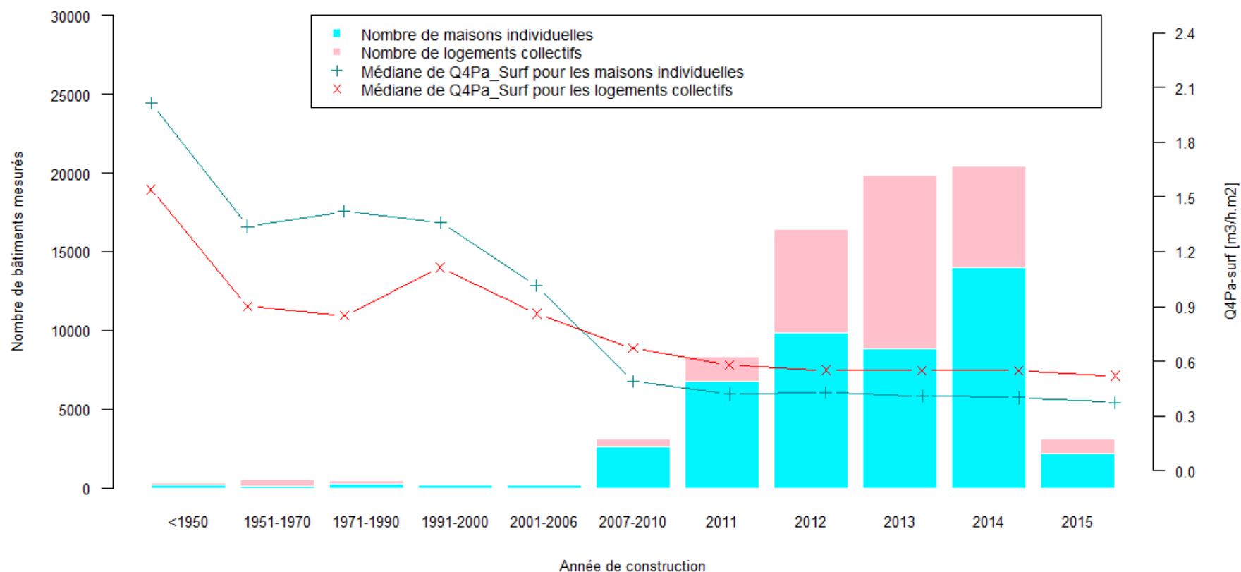
Evolution de la perméabilité à l'air des bâtiments résidentiels
