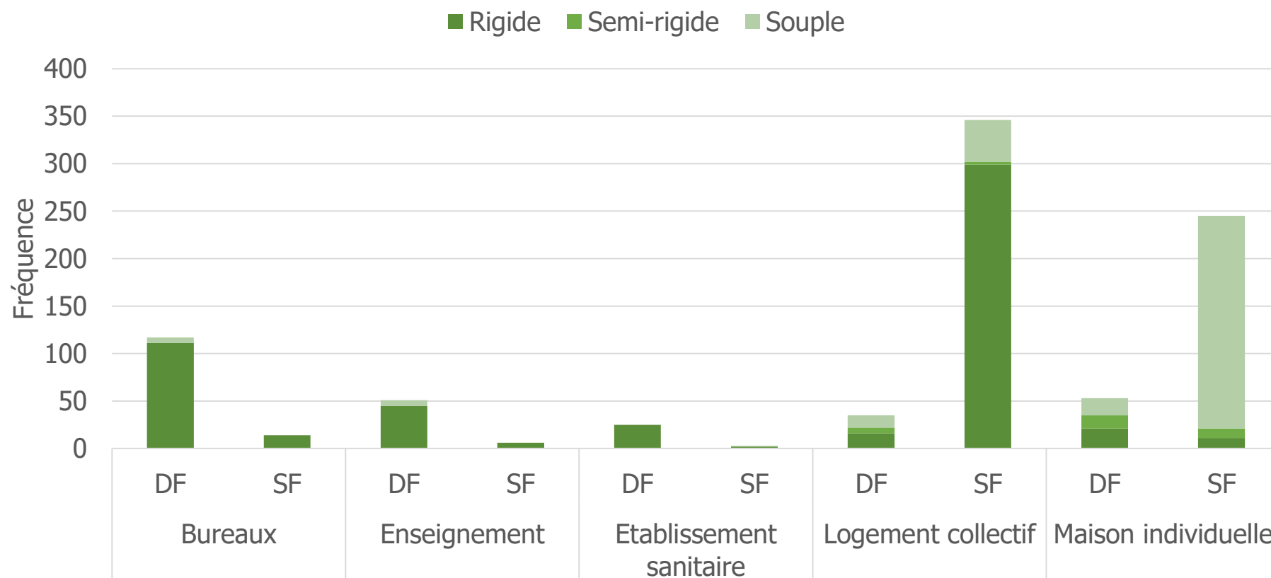
Répartition des mesures par système de ventilation et par type de réseau
